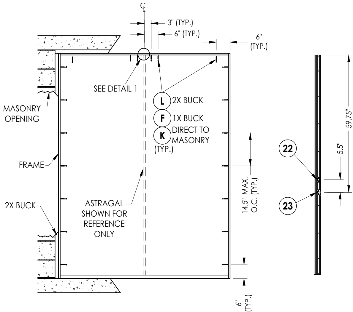
ASTRAGAL
