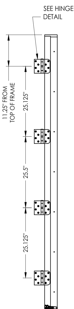
HINGE JAMB
